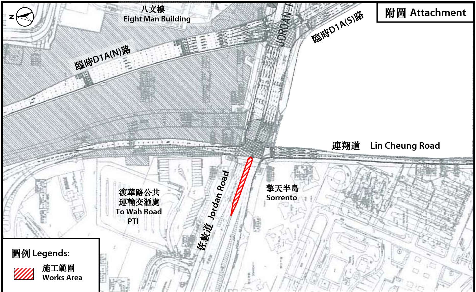
佐敦道臨時行人天橋橋墩建造工序 (由2011年12月7日、8日及9日, 凌晨1時至5時30分) Works for Temporary Footbridge Pier at Jordan Road (from 1:00am to 5:30am, 7 th , 8 th and 9 th December 2011)
