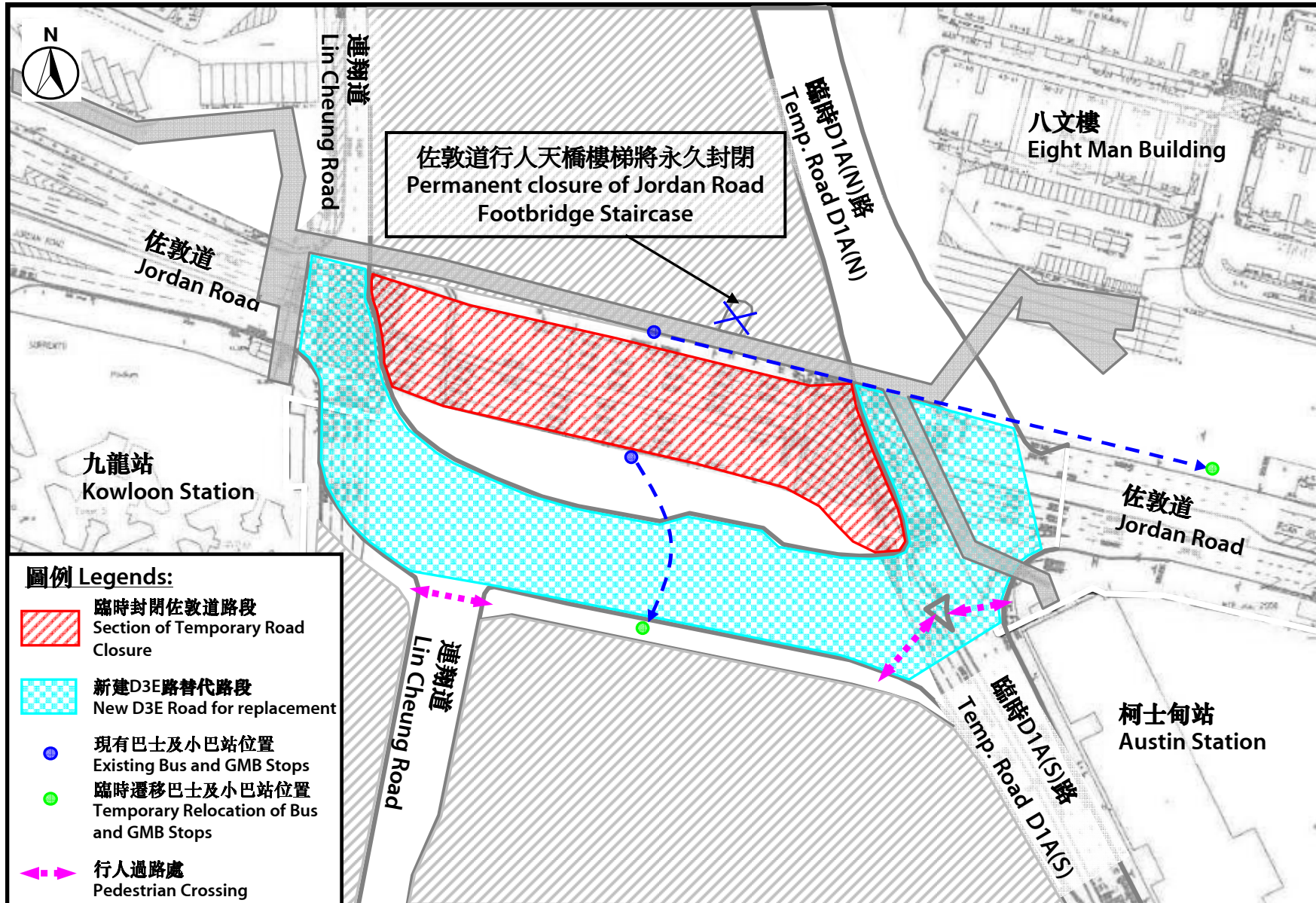
佐敦道之臨時交通管理措施 (2012年2月12日至2012年第三季) Temporary Traffic Arrangement for Jordan Road (From 12 February 2012 to Q3 of 2012)
